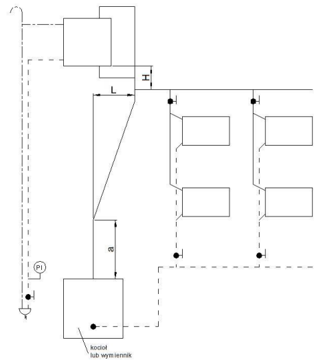
Wariant 1 - rozdział górny
