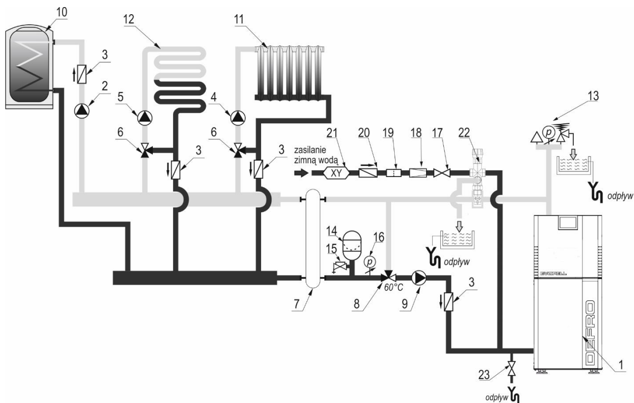
Rysunek 9. Uproszczony schemat instalacji grzewczej systemu zamkniętego.
