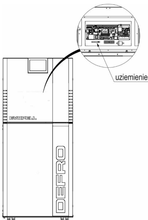
Rysunek 10. Uziemienie kotła.
