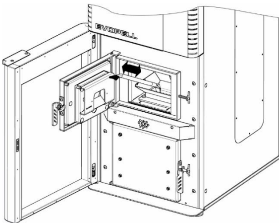
Rysunek 12. Sposób czyszczenia paleniska pelletowego.
