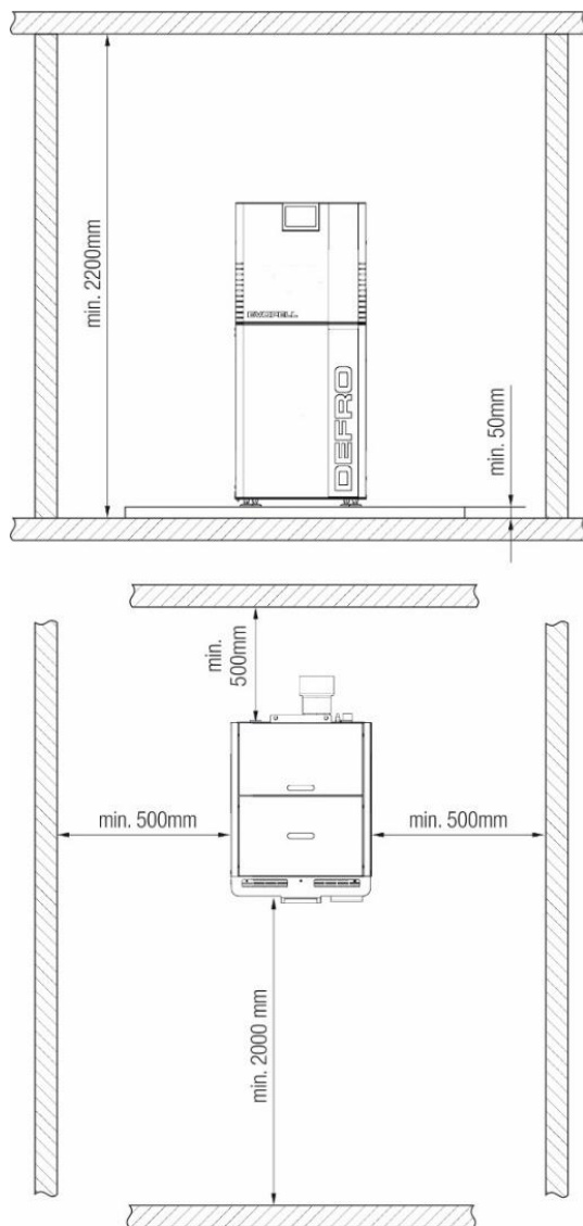
Rysunek 3. Ustawienie kotła w pomieszczeniu kotłowni.
