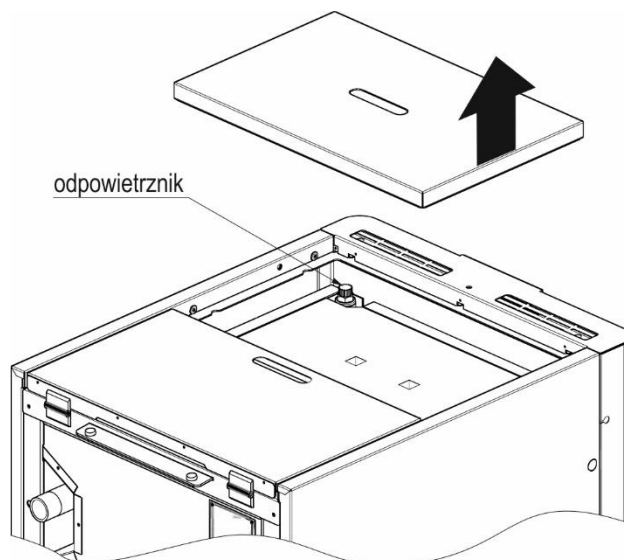
Rysunek 7. Odpowietrznik kotła.
