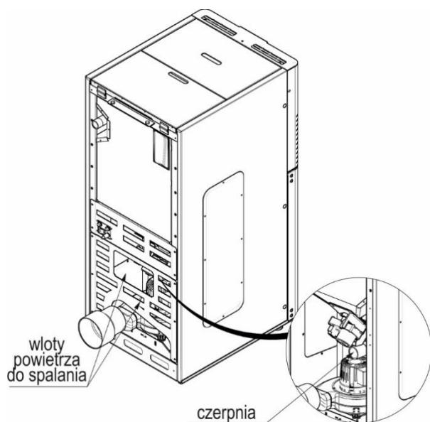
Rysunek 11. Czepnia powietrza - otwór dolotowy powietrza.
