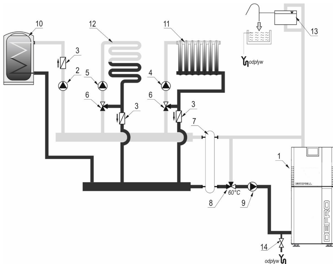
Rysunek 8. Uproszczony schemat instalacji grzewczej systemu otwartego.
