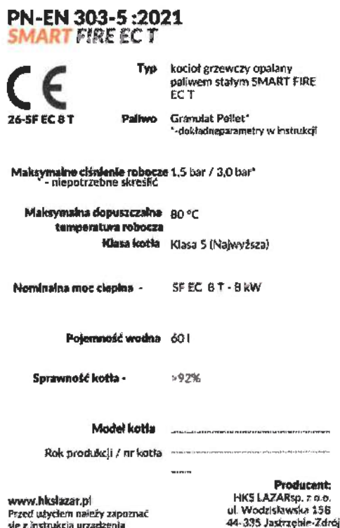
Rysunek 2. Tabliczka znamionowa kotła Smart Fire EC 8 T
