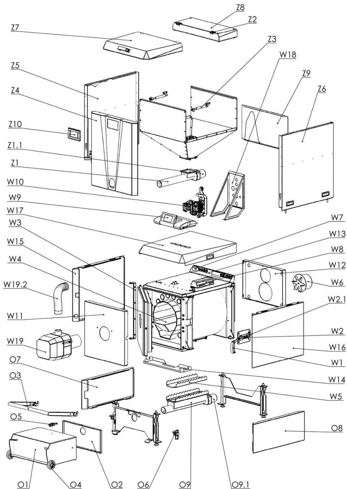
Rysunek 35 – Klasyfikacja części kotła
