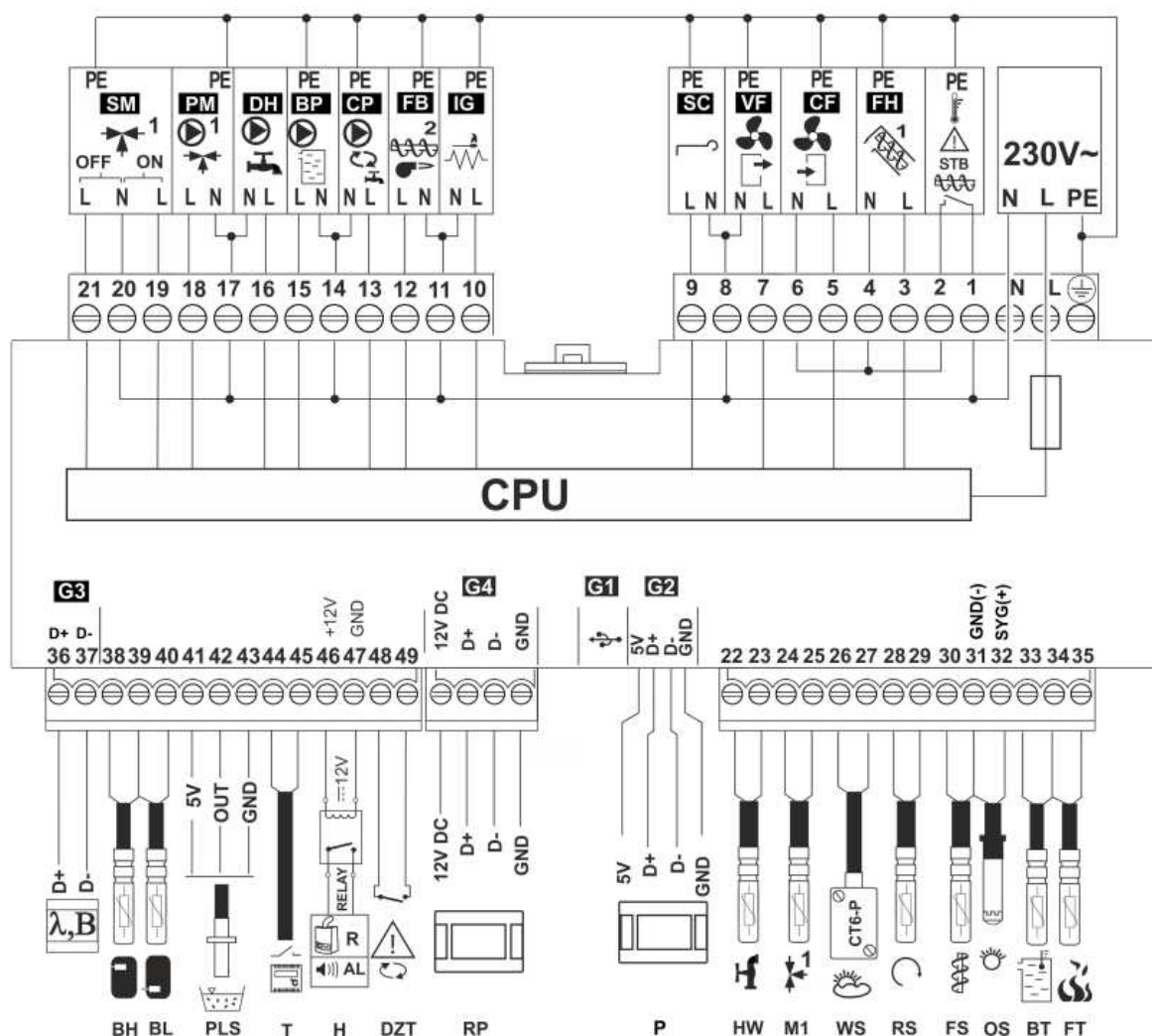
Rysunek 25 - Schemat połączeń elektrycznych regulatora: λ – moduł sondy Lambda, B – moduł do obsługi dodatkowych obiegów grzewczych, BH – czujnik temperatury bufora górny typu CT4, BL – czujnik temperatury bufora dolny typu CT4, PLS – czujnik poziomu paliwa, T – termostat pokojowy (zwierno-rozwierny), H – wyjście napięciowe do sterowania kotłem rezerwowym R lub do sygnalizacji alarmów AL , RELAY – przekaźnik 12VDC, DZT – czujnik otwarcia drzwi kotła, RP – panel pokojowy ecoSTER TOUCH z funkcją termostatu pokojowego, P – panel sterujący, HW – czujnik temperatury CWU typu CT4, M1 – czujnik temperatury obiegu regulowanego (mieszacza 1) typu CT4, WS – pogodowy czujnik temperatury typu CT6-P, RS – czujnik temperatury wody powracającej do kotła typu CT4, FS – czujnik temperatury podajnika typu CT4, OS – optyczny czujnik jasności płomienia, BT – czujnik temperatury kotła typu CT4, FT – czujnik temperatury spalin typu CT2S, L N PE – zasilanie sieciowe 230V~, CPU – sterowanie, STB – wejście do ogranicznika temperatury bezpieczeństwa, FH – podajnik główny, CF – wentylator nadmuchowy palnika, VF – wentylator wyciągowy, SC – silnik obrotowy czyszczenia palnika, IG – zapalarka, FB – podajnik palnika, CP – pompa cyrkulacji CWU, BP – pompa kotła, DH – pompa CWU, PM – pompa mieszacza 1, SM – siłownik mieszacza 1.
