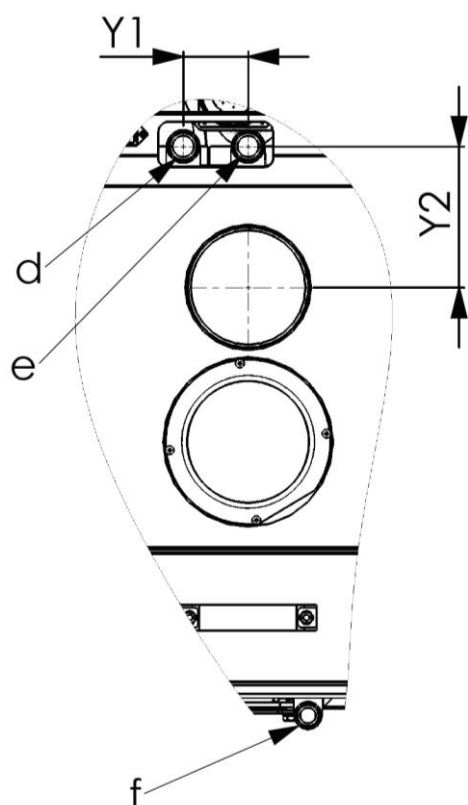
Rysunek 17 - Krocce podłączenia kotła do instalacji
