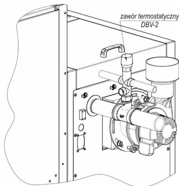
Rysunek 9. Przykładowy sposób podłączenia zaworu DBV-2.
