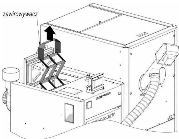
Rysunek 14. Sposób czyszczenia zawirówyacza.
