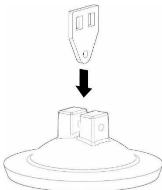
KROK 1. Wsunąć zawiesz deflektora w szczelinę.
