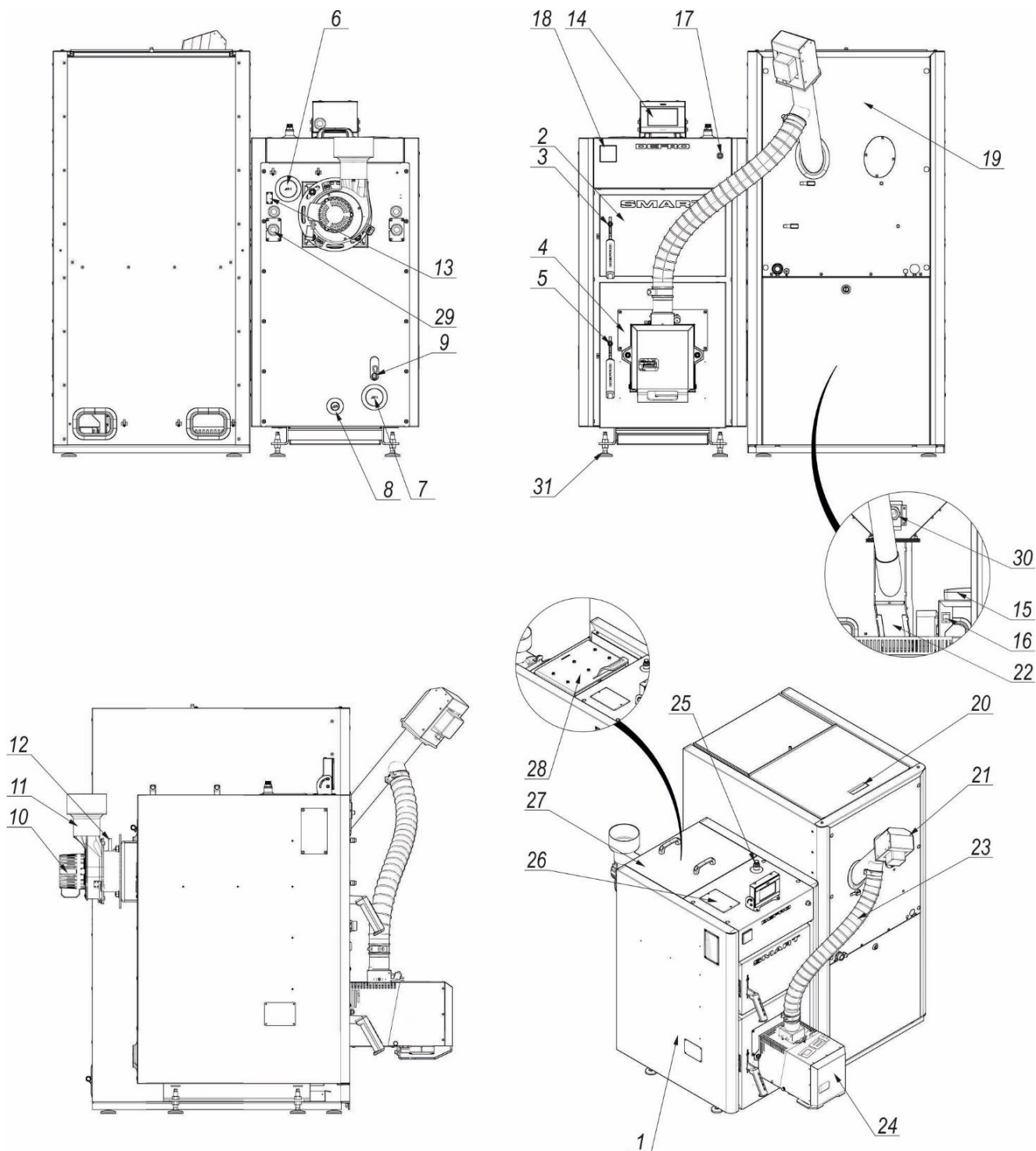
Rysunek 2. Podstawowe elementy kotła SMART EKOPELL.
