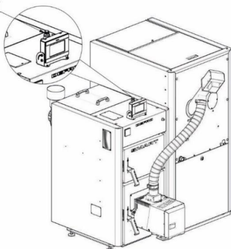
Rysunek 10. Odpowietrznik kotła
