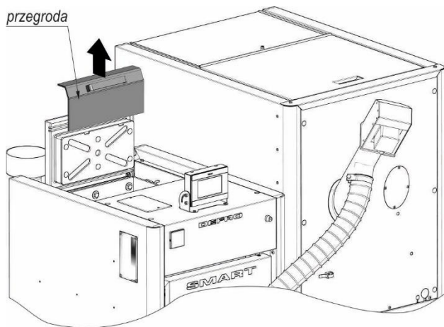
Rysunek 15 Sposób usunięcia przegrody
