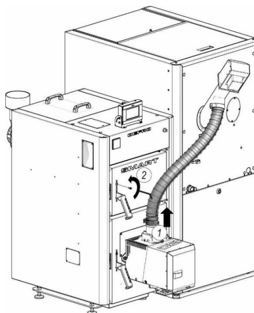
KROK 4. W celu zamontowania deflektora wewnątrz wymiennika należy zdemonstrować elastyczną rurę zsypu paliwa (1) i odkręcić śrubę zabezpieczającą drzwi wyczystne (2)
