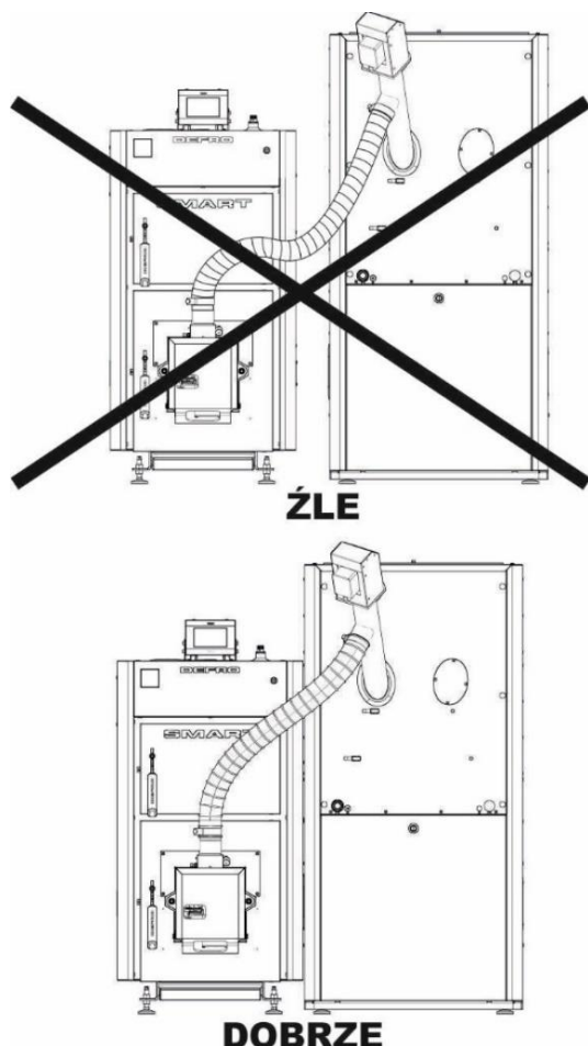
Rysunek 6. Prawidłowe ustawienie zasobnika paliwa względem kotła.
