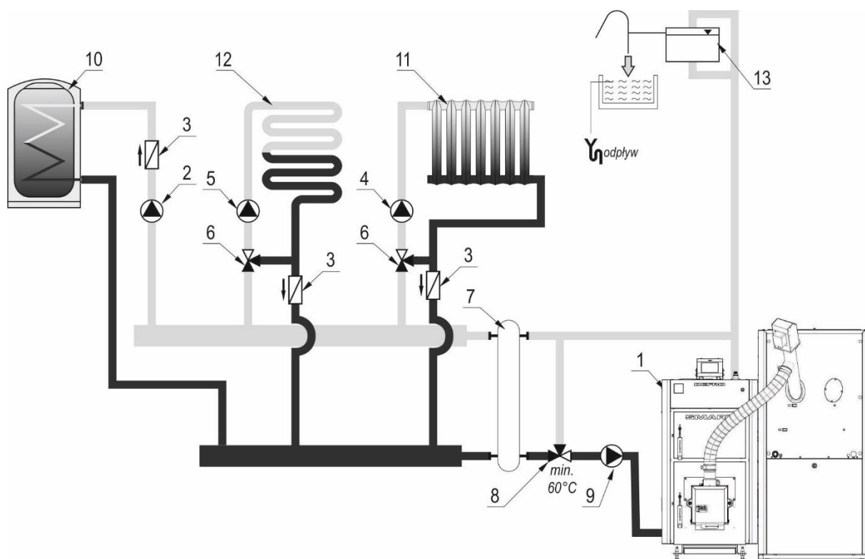
Rysunek 11. Uproszczony schemat instalacji grzewczej systemu otwartego.
