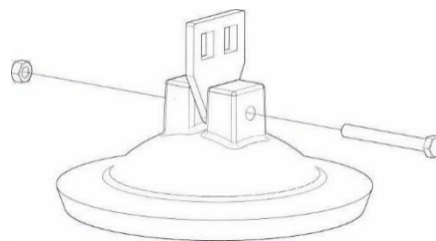
KROK 2. Zamocować zawiesz za pomocą śruby.
