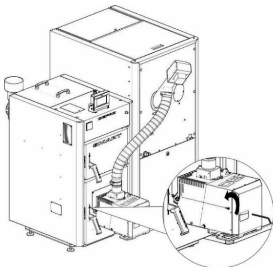
Rysunek 3. Sposób otwarcia drzwi kotła
