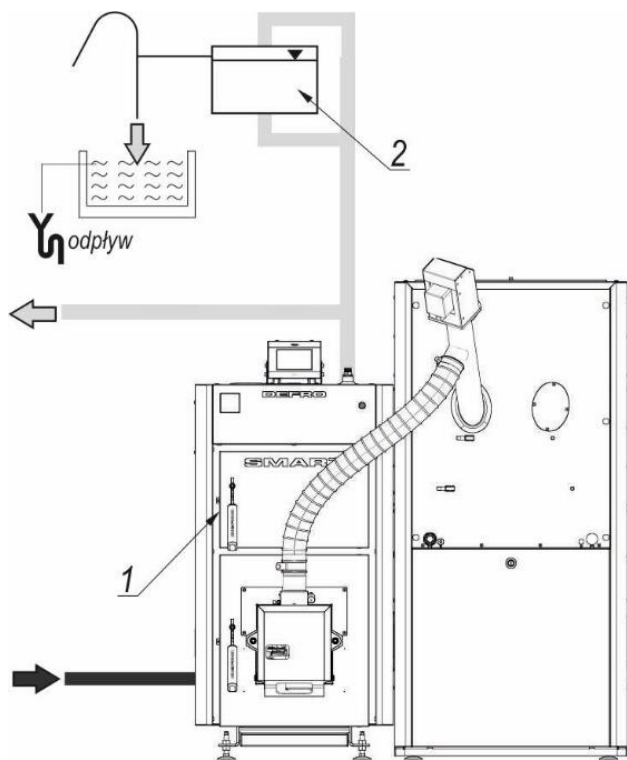
Rysunek 7. Przykładowy schemat zabezpieczeń kotła w układzie otwartym: 1-kocioł; 2-otwarte naczynie wzbiórcze.
