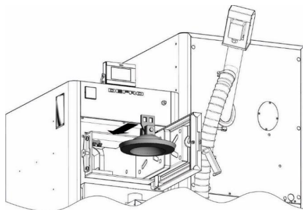
KROK 5. Otworzyć drzwi wyczystne oraz drzwi odbojnicowe i zawiesić deflektor na wieszaku. Następnie zamknąć drzwi i zabezpieczyć je śrubą zabezpieczającą
