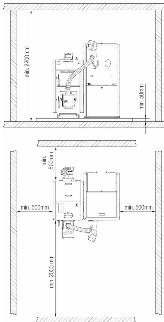
Rysunek 5. Ustawienie kotła w pomieszczeniu kotłowni.
