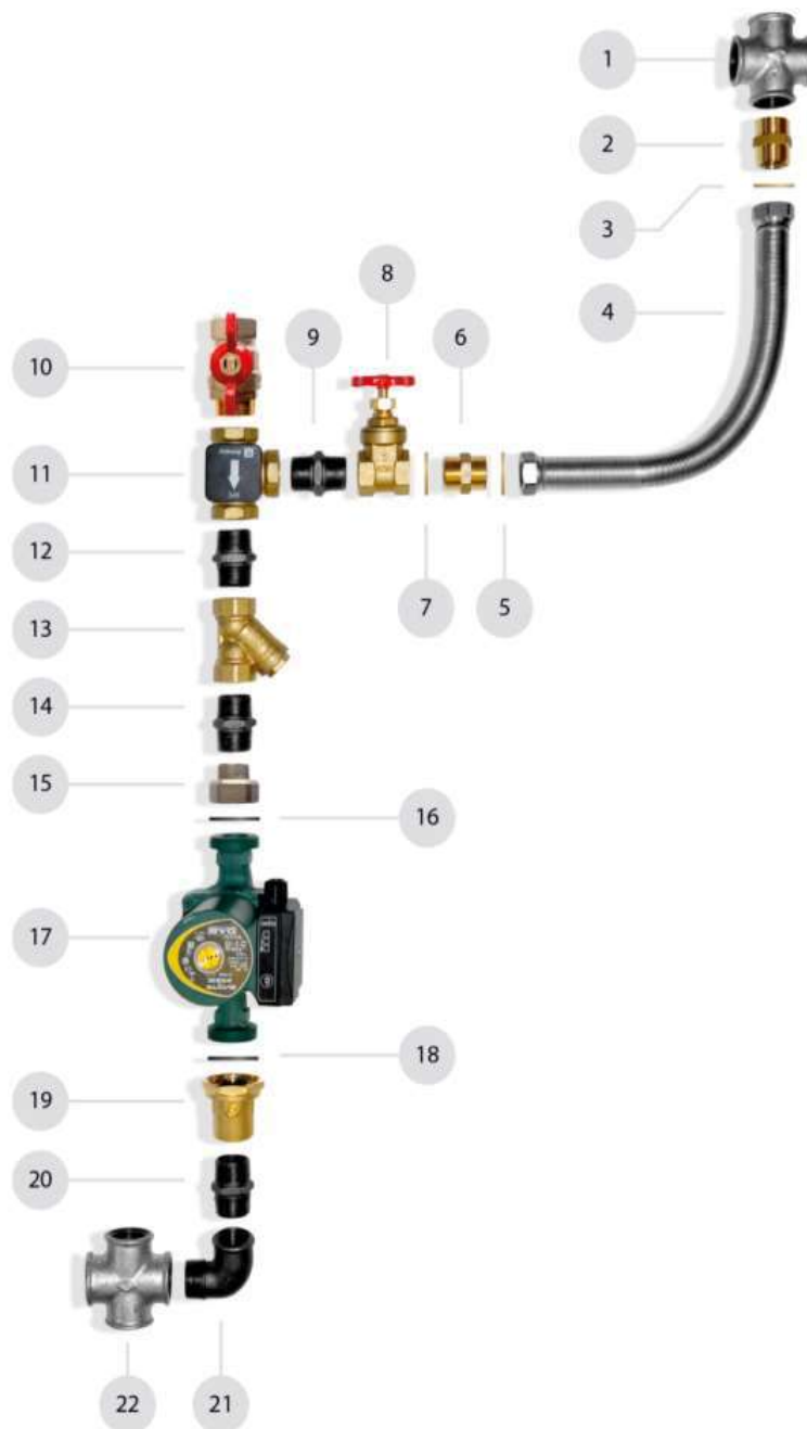
Rys nr 21. Zestaw hydrauliczny kotłów typu Smart Fire EC:
