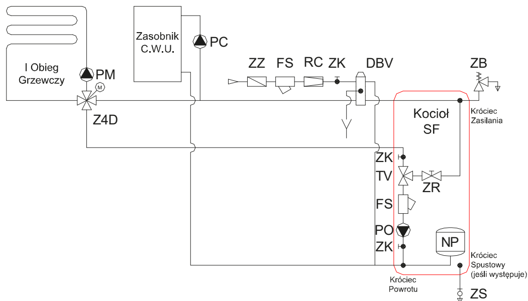
Rys nr 18. Układ zamknięty + CWU < 220 L + obieg na zaworze 4D
