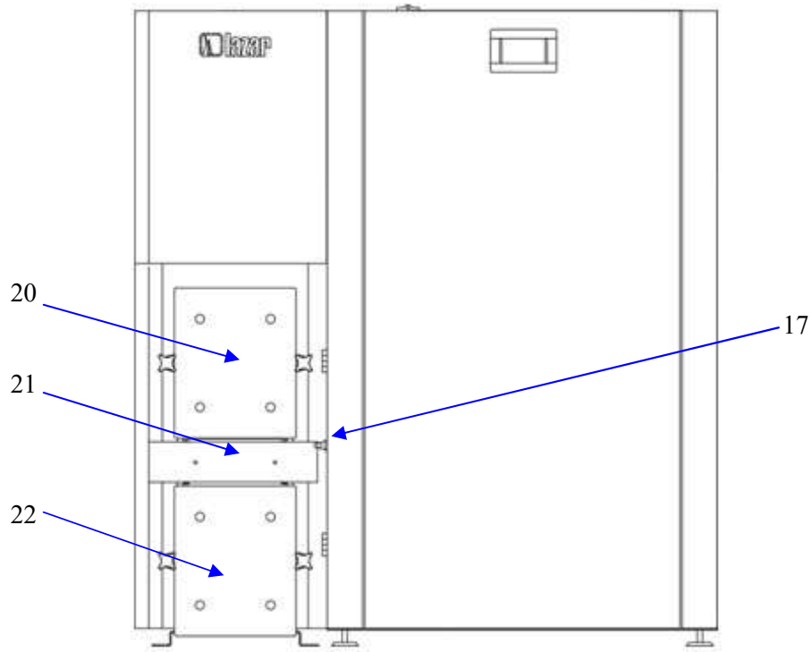
Rys nr 6. Opis schematyczny kotłów typu Smart Fire EC 15 oraz 21 17-wyłącznik krańcowy maskownicy drzwi kotła; 20-drzwi komory palnika; 21-maskownica zapalarki ceramicznej oraz wyczystki palnika; 22- drzwi komory popielnika;
