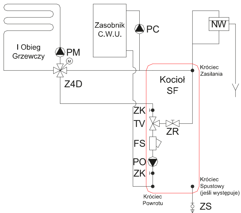
Rys nr 17. Układ otwarty + CWU<220L 1 obieg na zaworze 4D
