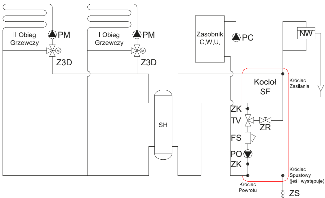
Rys nr 19. Układ otwarty + CWU < 220L + 2 obiegi na zaworze 3D
