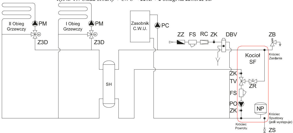
Rys nr 20. Układ zamknięty + CWU < 220L + 2 obiegi na zaworze 3D
