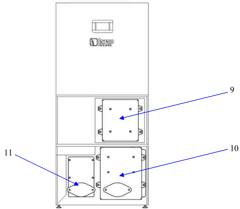
Rys nr 10. Opis schematyczny kotłów typu Smart Fire EC T: 9- drzwi komory spalania; 10-drzwi komory popielnika; 11 – wyczystka dolnej części wymiennika ciepła
