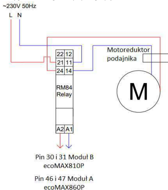
Rys nr 12. Schemat podłączenia systemu automatycznego odpopielania do regulatora kotła.
