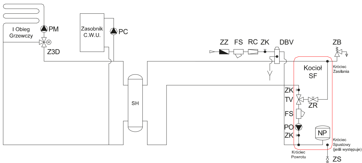
Rys nr 15. Układ zamknięty + CWU > 220L + 1 obieg na zaworze 3D
