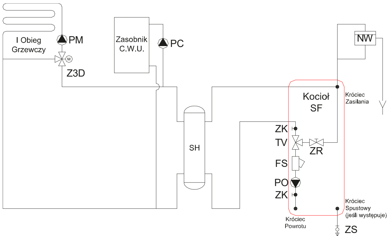
Rys nr 14. Układ otwarty + CWU > 220L + 1 obieg na zaworze 3D
