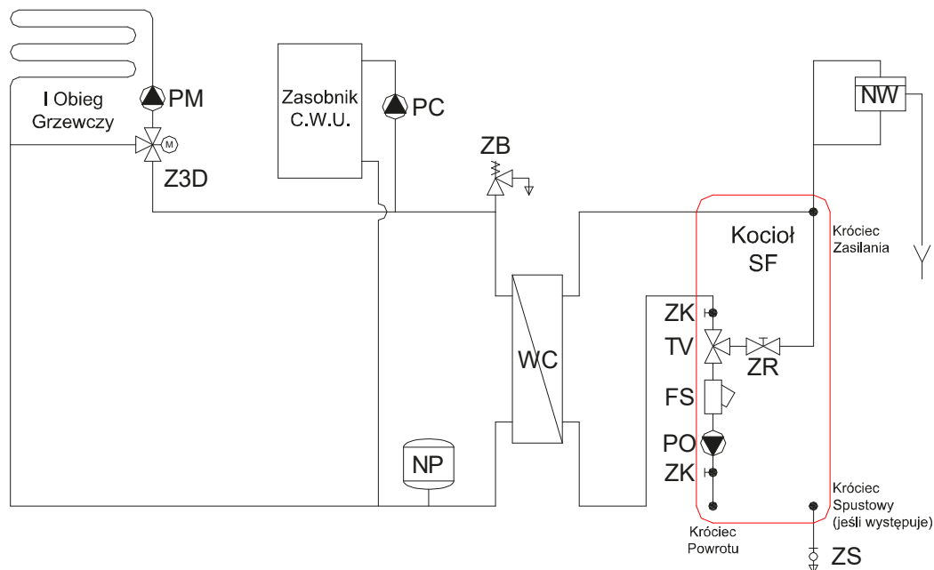
Rys nr 16. Układ z płytowym wymiennikiem ciepła – kocioł w układzie otwartym, wymiennik CWU i obieg grzewczy w układzie zamkniętym
