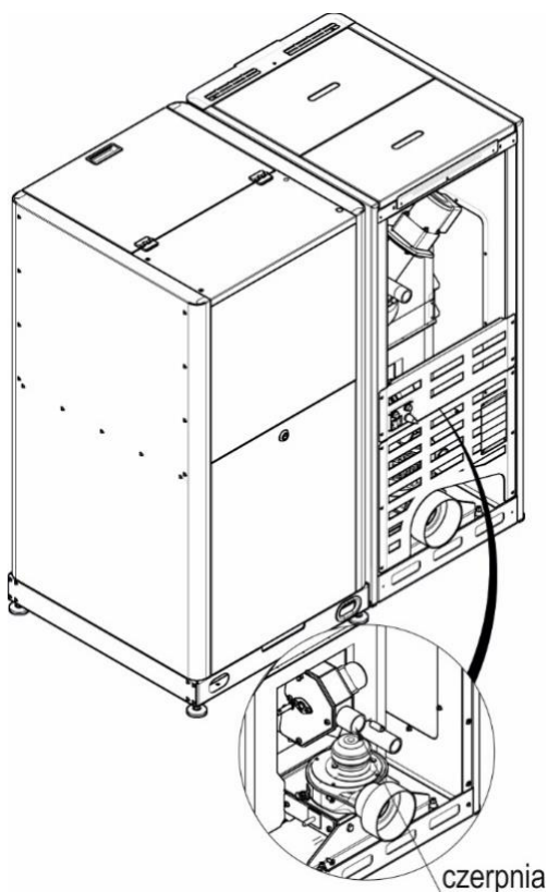
Rysunek 13. Czerpnia powietrza - otwór dolotowy powietrza.
