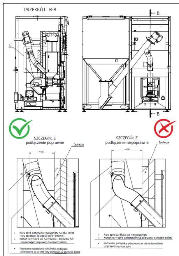
Rysunek 5. Ułożenie rury spiro zsypu paliwa
