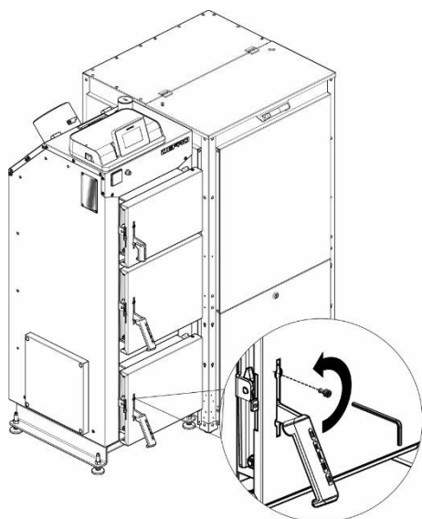
Rysunek 3. Sposób otwarcia drzwi kotła
