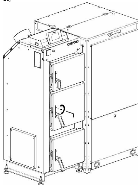
KROK 1. Odkręcić śrubę zabezpieczającą drzwi paleniskowe
