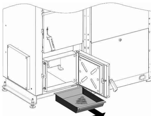
Rysunek 11. Szuflada na popiół
