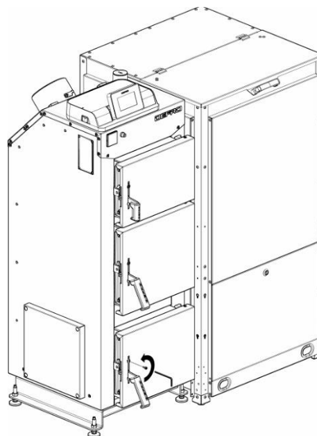
KROK 1. Odkręcić śrubę zabezpieczającą i otworzyć drzwi popielnikowe kotła.
