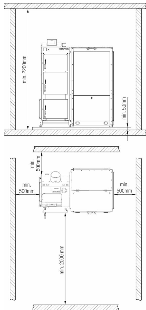
Rysunek 5. Ustawienie kotła w pomieszczeniu kotłowni.
