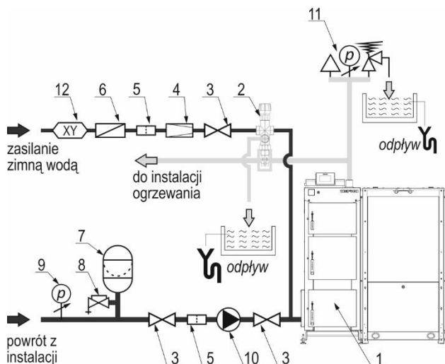
Rysunek 7. Przykładowy schemat zabezpieczeń kotła KOMFORT EKOPELL w układzie zamkniętym
