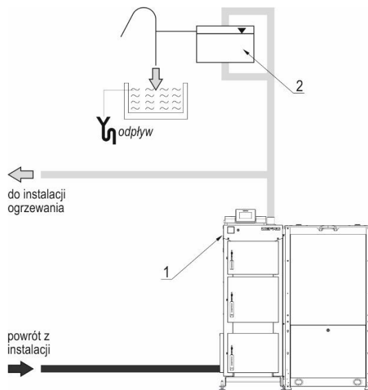
Rysunek 6. Przykładowy schemat zabezpieczeń kotła KOMFORT EKOPELL w układzie otwartym
