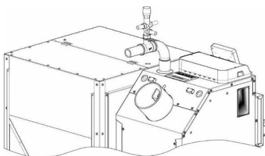
Rysunek 8. Przykładowy sposób podłączenia zaworu DBV-2.
